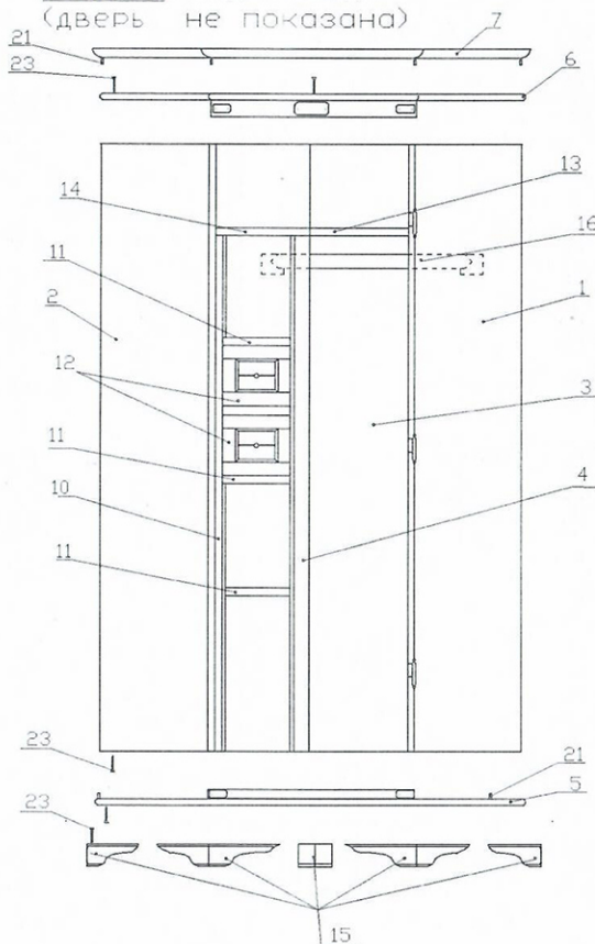
Схема 2. Вид фасада (дверь не показана)
